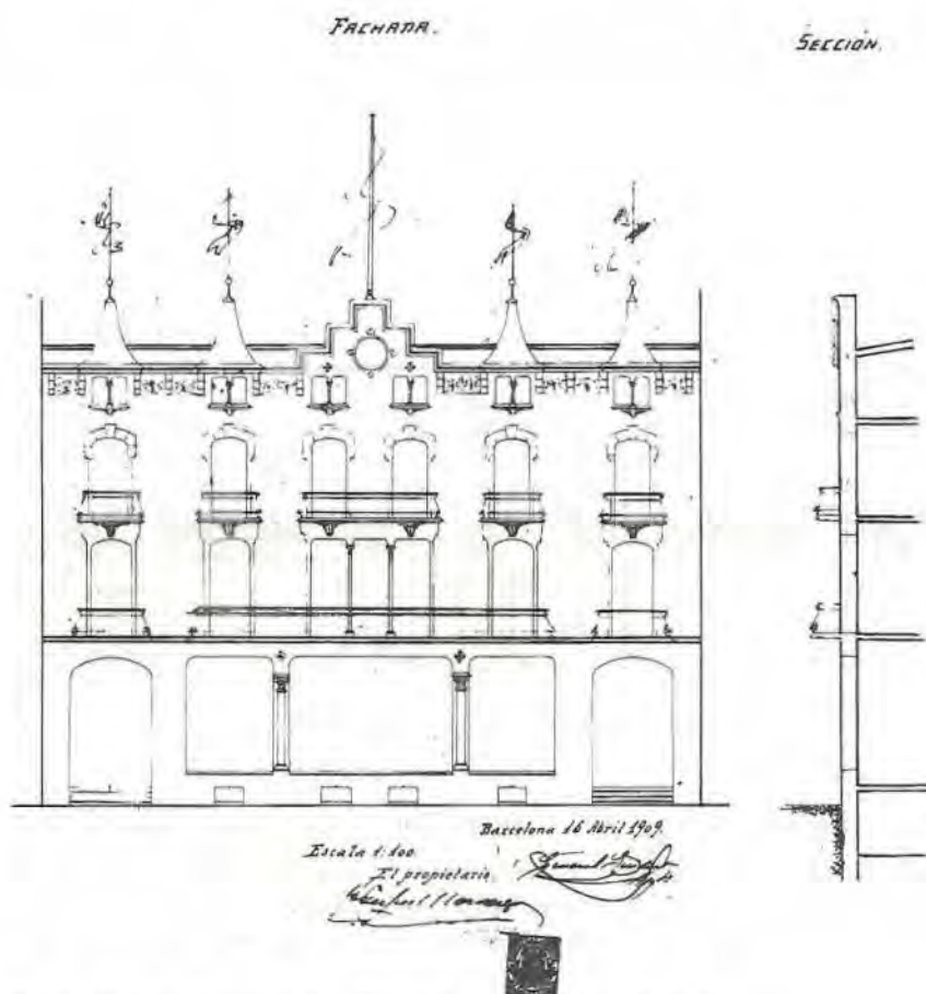
Fig. 4. Projecte del casino dels "Senyors" o "El Guixolense", 1909.
