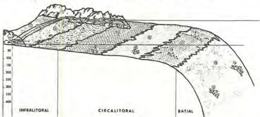
Figura 1. Esquema de la successió de plans a la plataforma continental. 1) Massa rocosa. 2) Detritus al·luvials. 3) Plans supralitoral i mesolitoral. 4) Sorres fines, poc fondes. 5) Sorres fines, de més fondària. 6) Roques de la zona infralitoral. 7) Praderies de Posidonia . 8) Zones coral·lígenes. 9) Fons de detritus costers. 10) Fangs terrígens costers. 11) Fons detritics litorals. 12) Fons batials. 13) Corals de profunditat. (Segons G. Spada).
