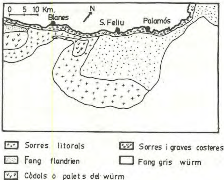
Figura 10. Morfologia del fons submarí de la zona sud. (Segons Serra).
