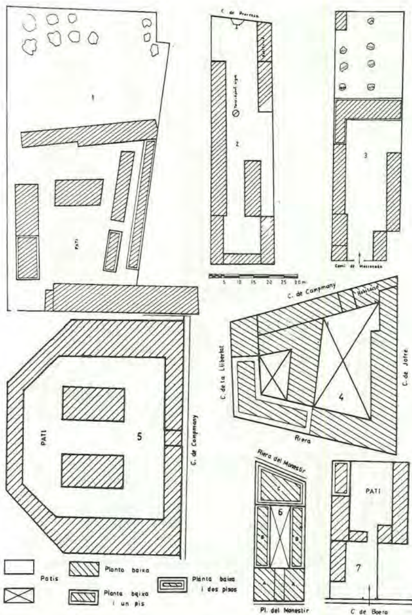
Fig. 1. Plans de les diverses fàbriques guixolenques. 1 (núm. 4 de Joan Bordás Fills de H. A. Bender. 2 (núm. 7 id Bombí i Soler. 3 (9 id Enric Rosselló. 4 (3 id Industrial Bolsera. 5 (2 id Banaset i Sanmiquel, 6 (1 id Josep Mont, 7 (8 id Llorenç Moner.
