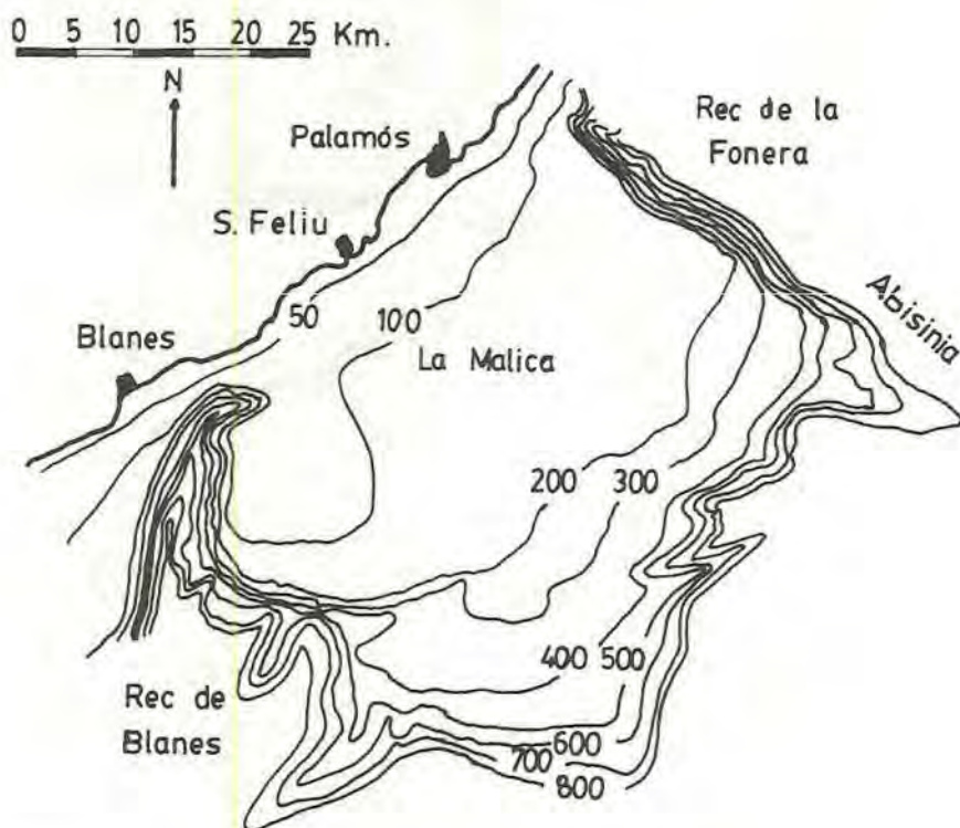
Figura 8. Relleu submarí de la zona sud; profunditats en metres.
