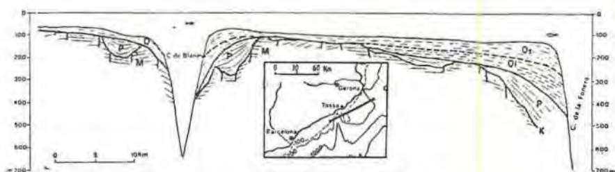
Figura 9. Tall geològic de la zona sud. (Segons Serra). M) Miocèn. P) Pliocèn, Qi) Quaternari inferior. Qs) Quaternari superior.
